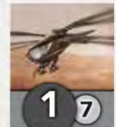
Ornithopter
